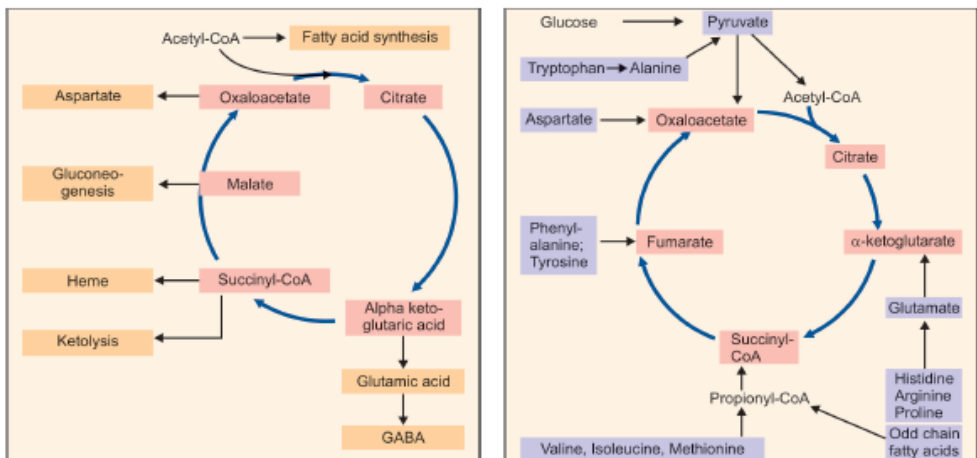
شکل (۴): کریب سیکل ته د کاربوني واحدونو داخلیدل او خارجیدل
