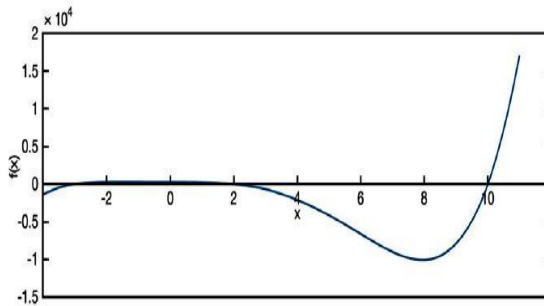
۱ شکل نوموړی گراف په لومړي مثال کې f(x) تشریح کوي.
