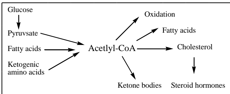
(۱) شکل: د اسیتایل کوانزیم ای منابع او د استعمال لوري
