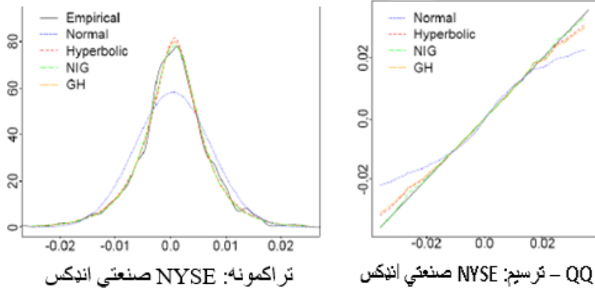
(۱- شکل): د تراکم او QQ-plot د مختلفو توزیع گانو په برابری کې لوگاریمي خروجي ته په ورکولو سره د NYSE شاخص رابښي. (۲ جون ۱۹۹۰ څخه تر ۱۱ نومبر ۱۹۹۶) (۹، ص ۲۰۰-۲۳۴)
