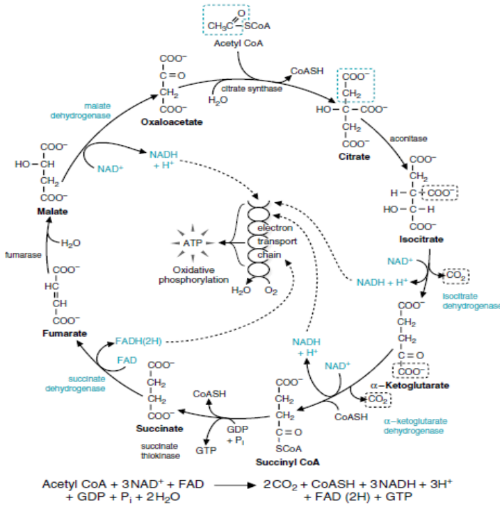
شکل (۳): د کریب سیکل (تراي کاربوکسلیک اسید سیکل) یا دسیتریک اسید دوران د یوې دورې خلاصه
