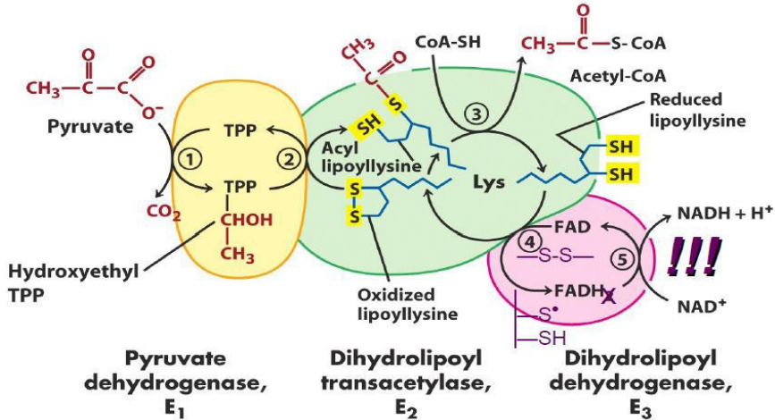
(۲) شکل: د پایرویت بدلیدل په استیایل کوانزایم ای باندي
