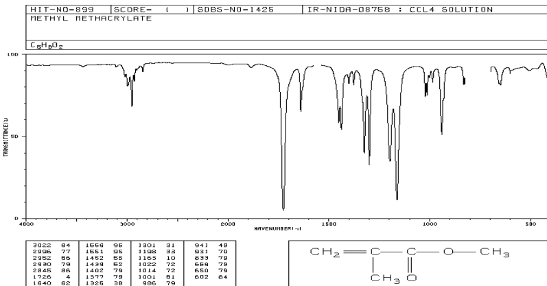
(۵) شکل: د میتایل میتا کریلات د FT-IR سپکټروسکوپي طيف
