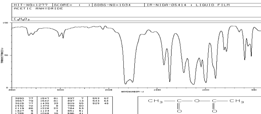
(۷) شکل د استیک اسید انهایدرايد د FT-IR سپکټروسکوپي طيف
