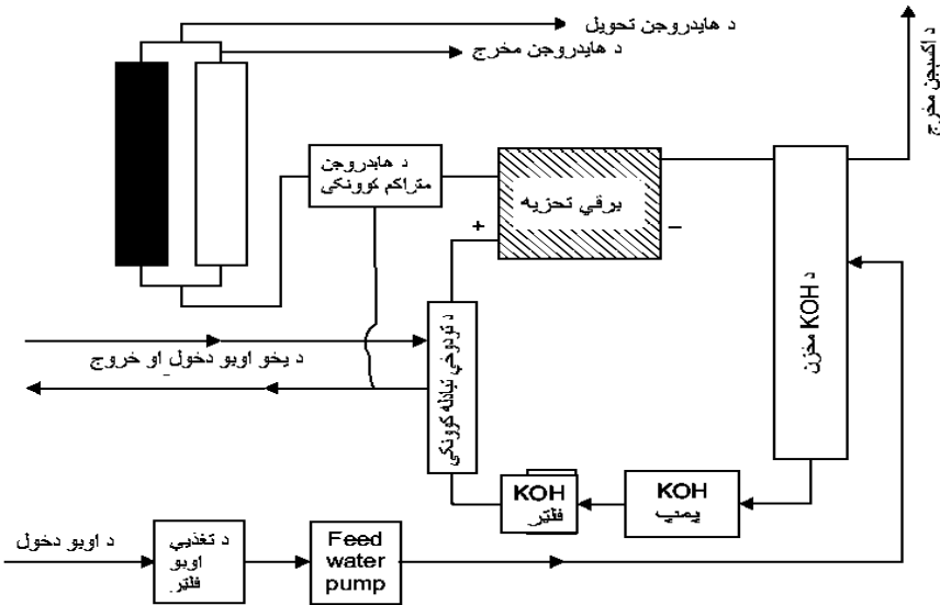
1- شکل: د القلي د برېښنايي تجزيې څخه د هایدروجن تولید. [3]
