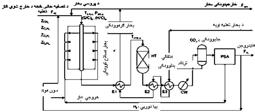
۲ - شکل: د هایدروجن د تولید د پروسې ساده شوی دیاگرام. [3]
