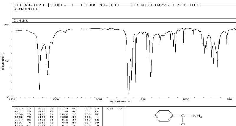
(۶) شکل: د بنزاماید د FT-IR سپکټروسکوپي طيف
